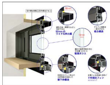
樹脂サッシの構造
